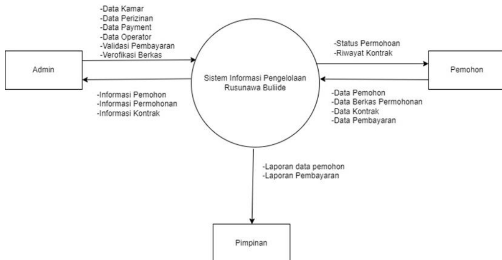
Gambar 3. Diagram Konteks
